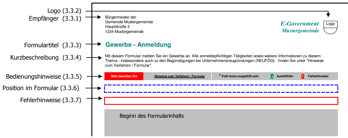
Abbildung 2: Kopfzeile der Formular-Startseite
